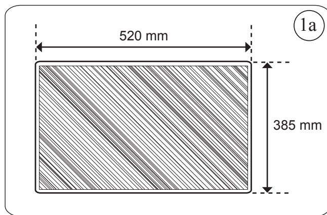
Dimensioni minime per il taglio sul tetto della cabina, se non dispone di un oblo'
