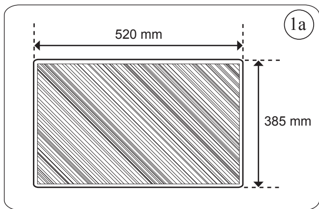
Dimensions min. de découpage du toit de la cabine s'il n'y a pas d'écoutille
